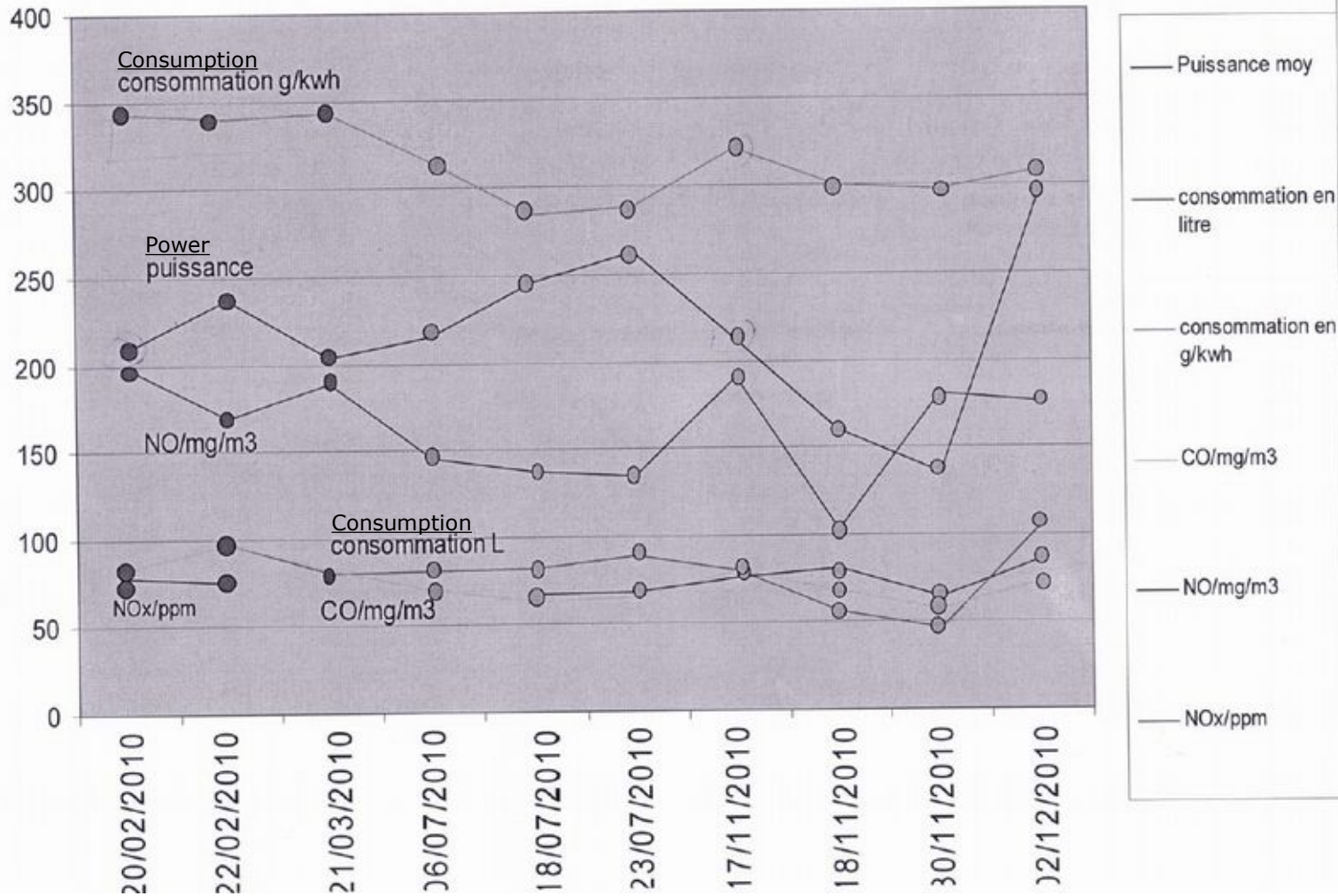
puissance; consommation L; consommation g/kwh CO/mg/m3; NO/mg/m3; NOx/ppm
